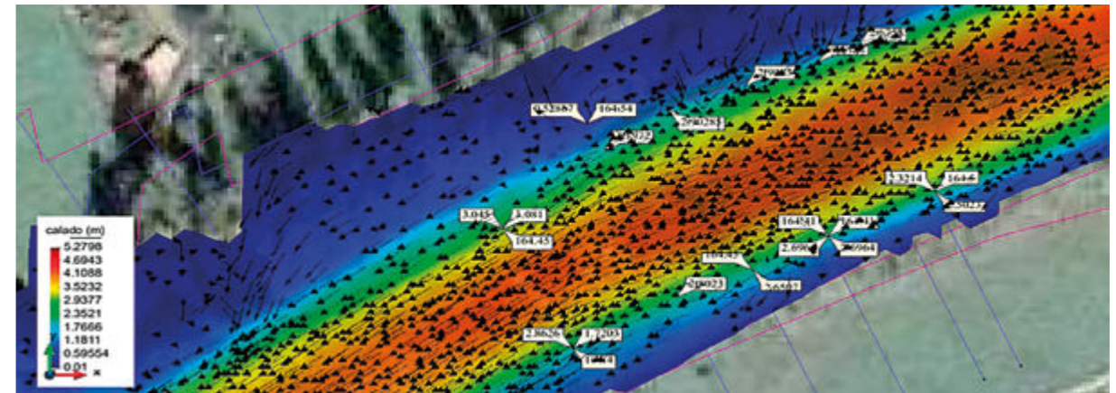
Ejemplo de simulación bidimensional realizada en el proyecto Arraioz. Fuente: SCIA SL
