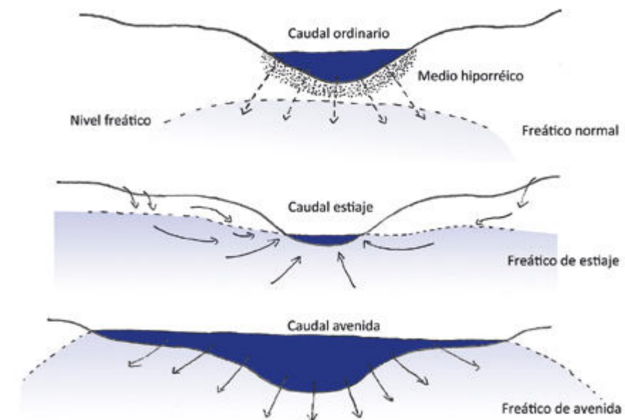
Dimensión vertical del río. Ilustración: S. Sangalli
