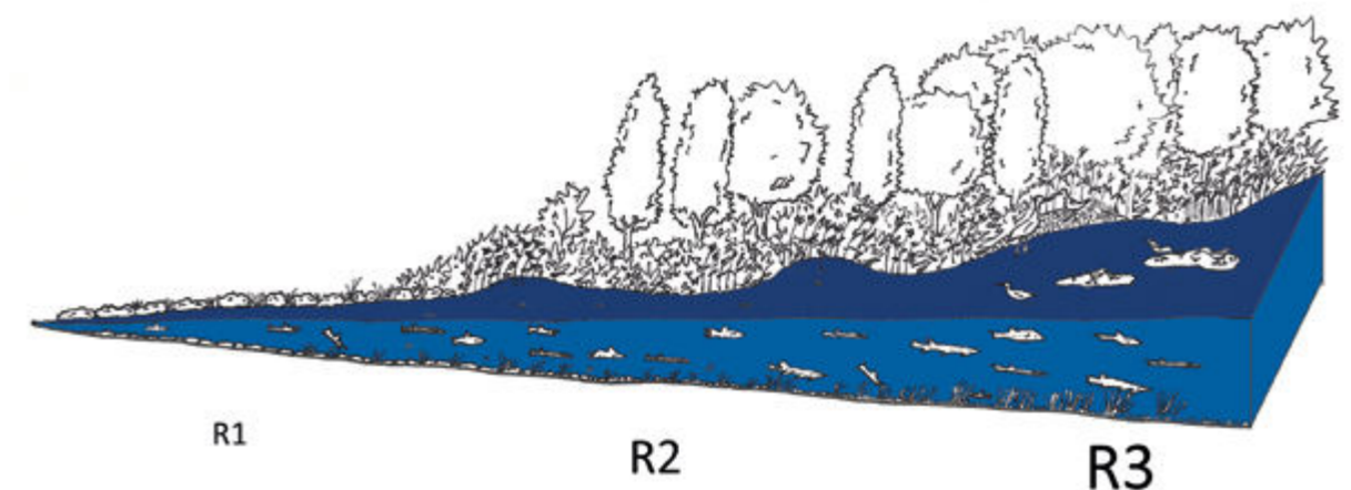
Factores generales de influencia en la biocenosis acuática y en la calidad ecológica general del curso fluvial. Fuente: Bernard Lachat
