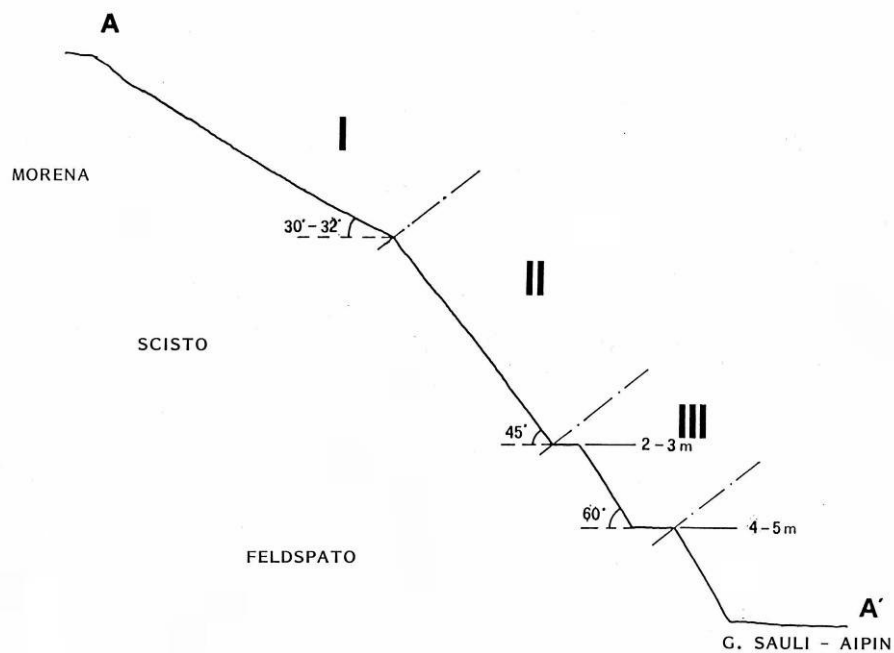
Profilo delle morfologie mineraria di feldspato di Giustino (TN)
